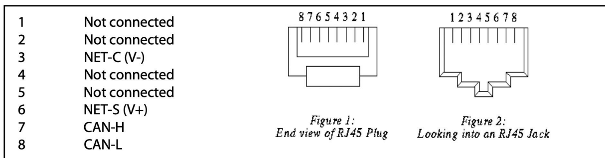
Victron VE.Can Pinbelegung
