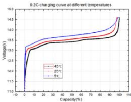
Unterschiedliche Temp. Ladungskurve (0,2C)
