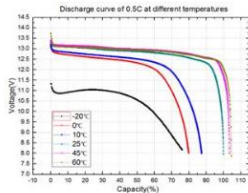
Unterschiedliche Temp. Entladungskurve (0,5C)
